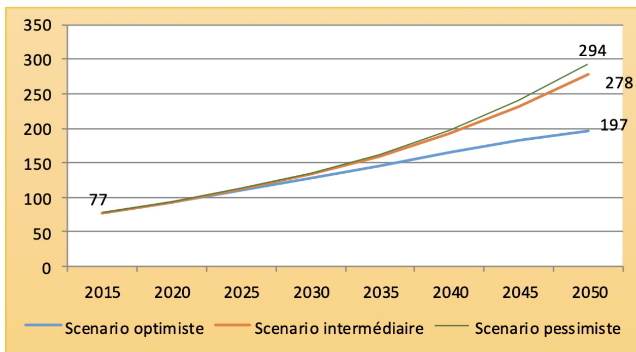
Figure 21. Projection de la population de la RDC en millions d'habitants à l'horizon 2050
