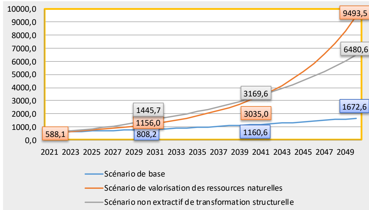
Figure 10. RDC, projections du PIB par habitant (en dollars US constants de 2021) à l'horizon 2050 en trois scénarios
