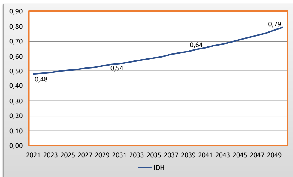
Figure 16. RDC, projections de l'IDH à l'horizon 2050 (échelle de 0 à 1, PNUD)
