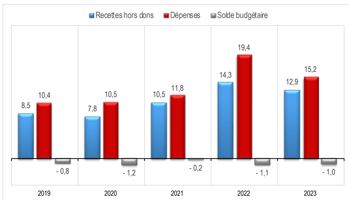
Figure 4. Évolution des finances publiques en % du PIB (2019-23)
