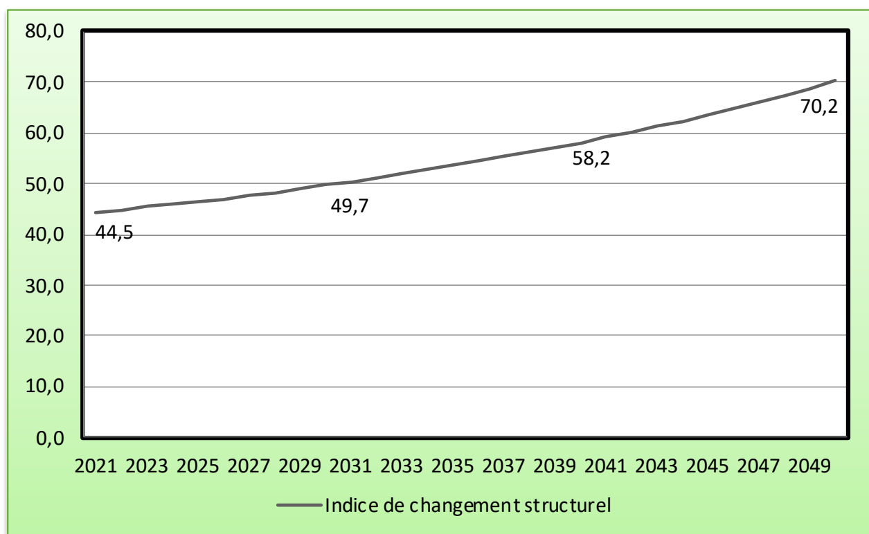
Figure 20. RDC, projections de l'indice de changement structurel (échelle de 1 à 100) sur l'horizon 2050
