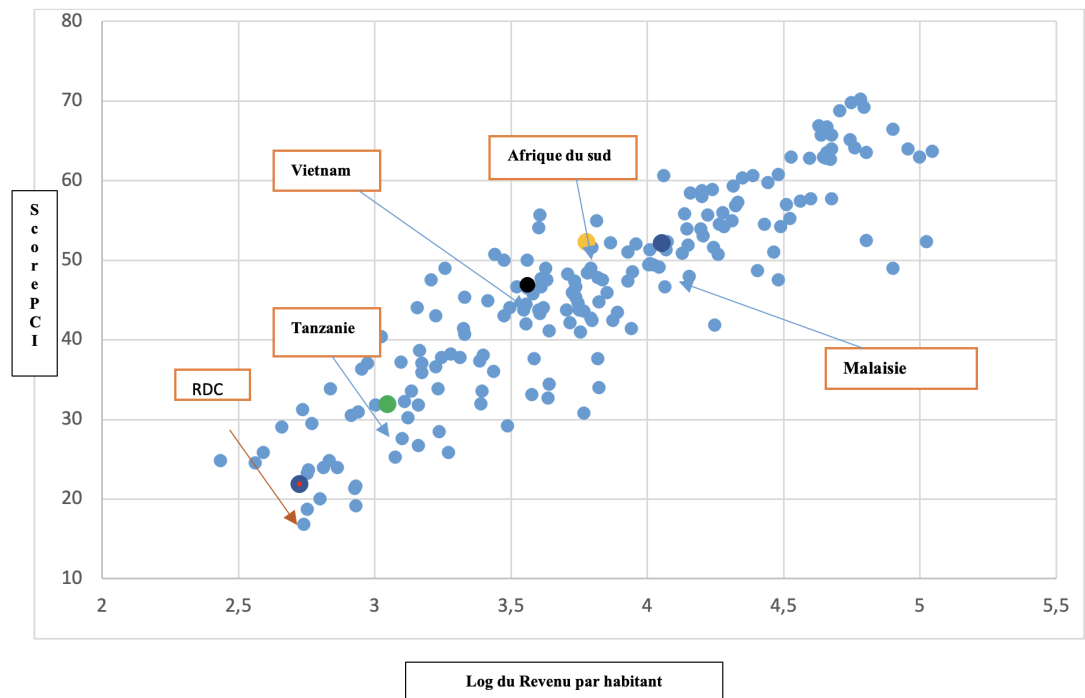
Figure 14. Corrélation entre le score PCI et le revenu par habitant
