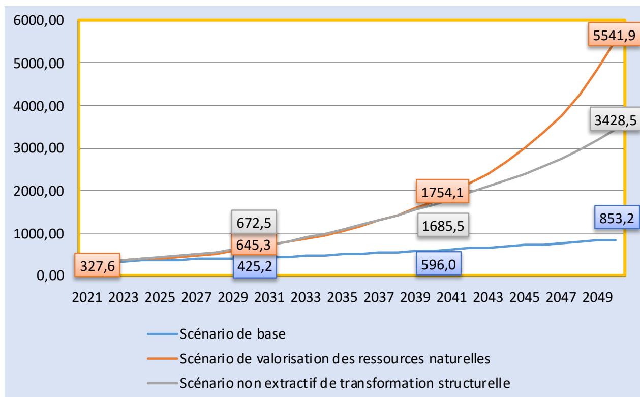
Figure 12. . RDC, projections de la valeur ajoutée manufacturière per capita (en dollars US constants de 2021) à l'horizon 2050 en trois scénarios
