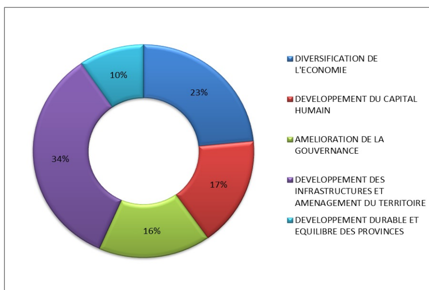
Figure 25. Part de chaque domaine dans le coût global du PNSD 2024-2028
