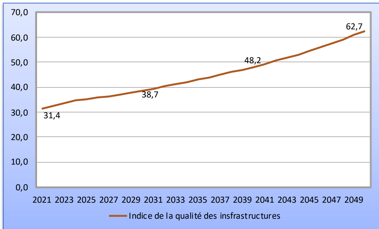
Figure 19. RDC, projections de l'indice de qualité des infrastructures (échelle de 0 à 100) à l'horizon 2050
