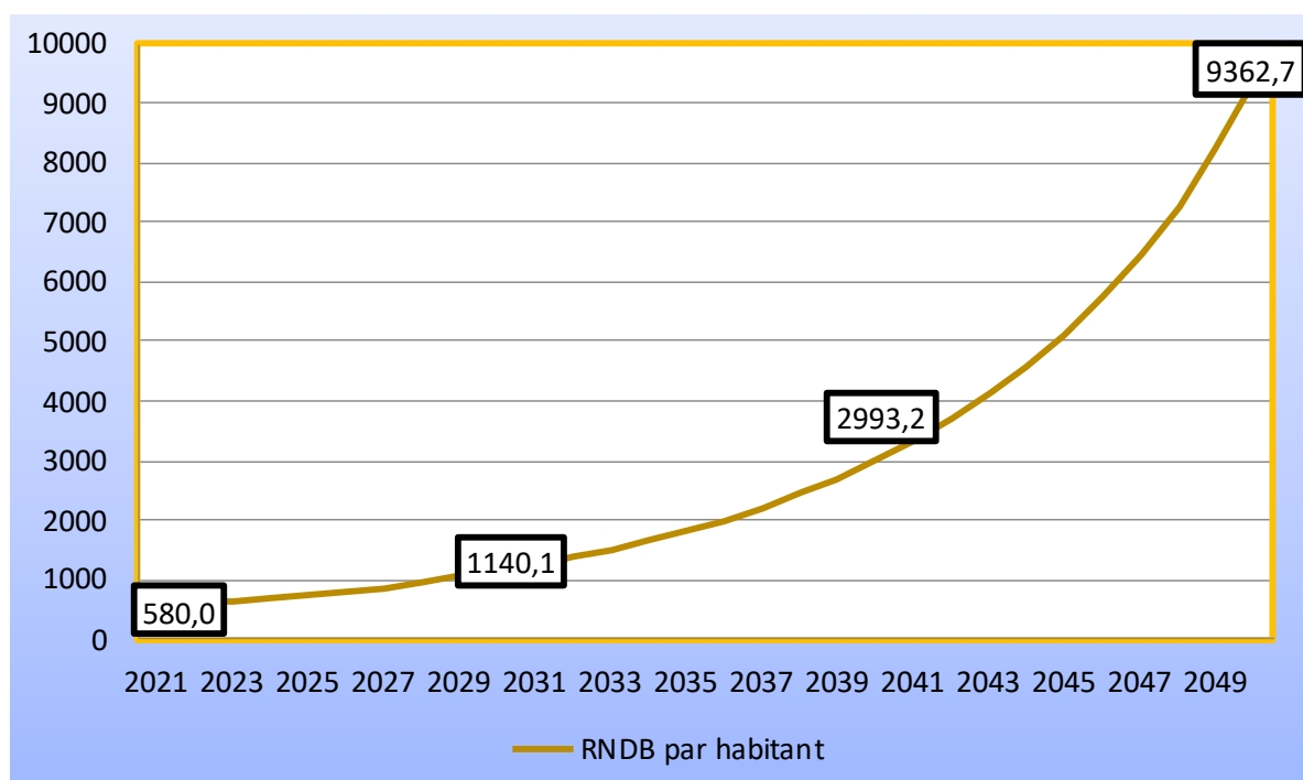
Figure 15. RDC, projections du RNDB par habitant à l'horizon 2050 (en USD constants de 2021)
