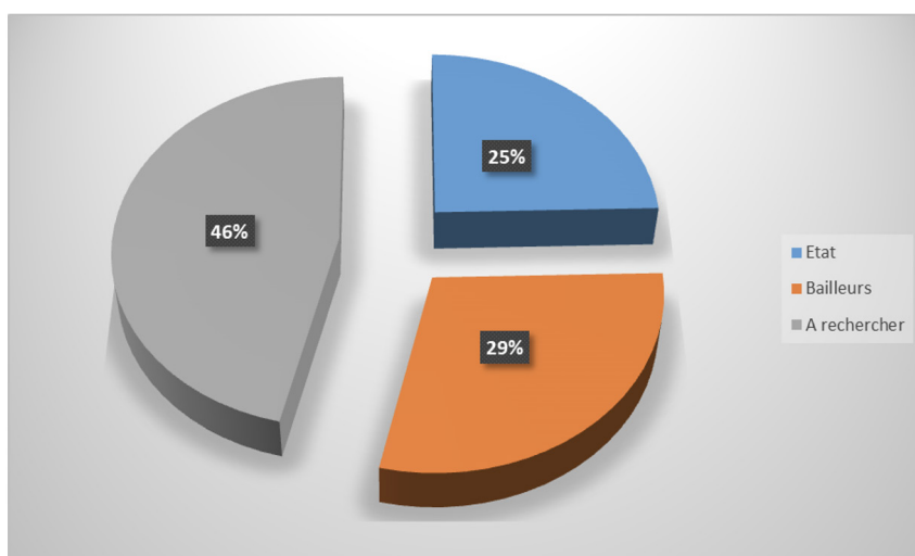
Figure 24. Répartition des besoins de financement de développement par source de financement des besoins d'investissement
