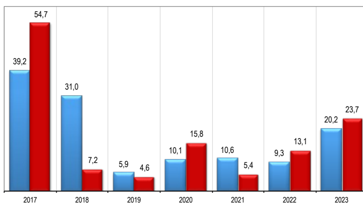
Figure 3. Évolution annuelle des taux d'inflation en pourcentage (2017-23)
