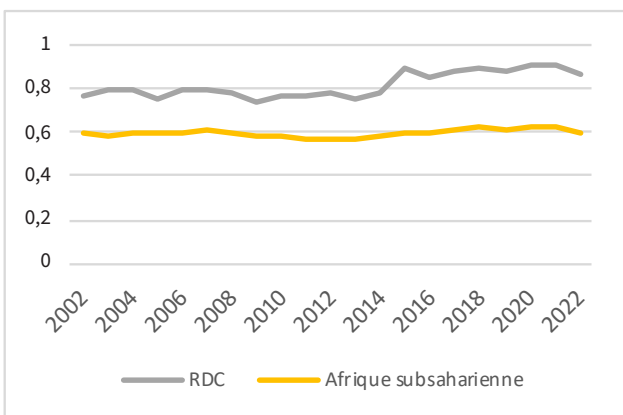
Figure 8b. Indice de dispersion : RDC et ASS, 2002-2022
