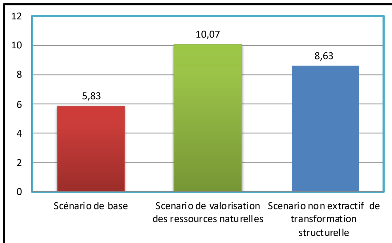
Figure 9. Croissance du PIB de la RDC (en %), moyenne annuelle, 2021-2050
