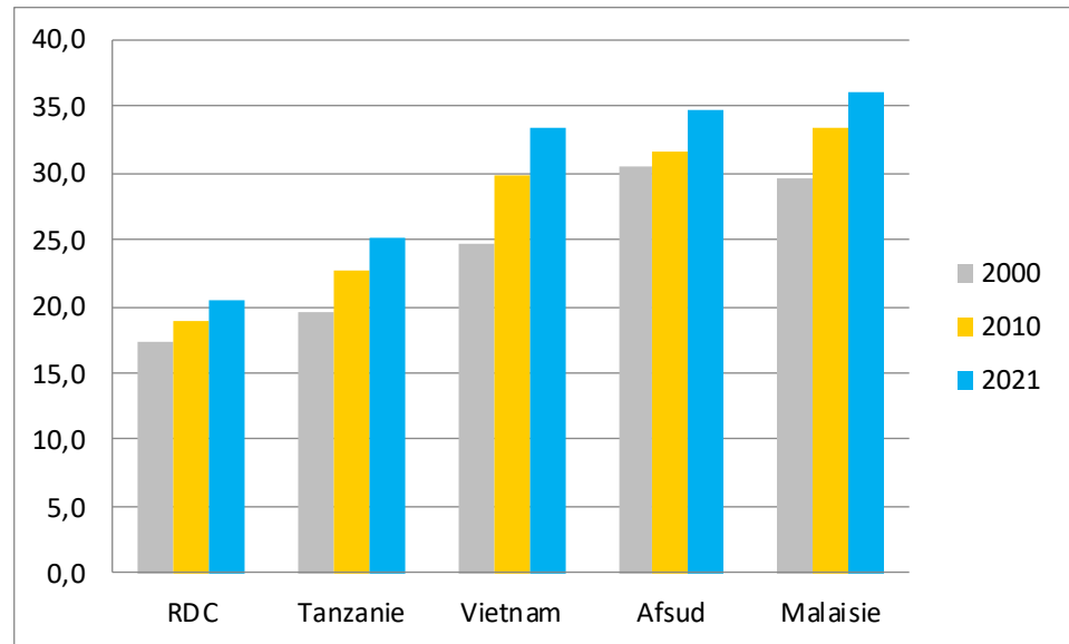
Figure 13. Capacités productives de la RDC et de quelques pays comparateurs
