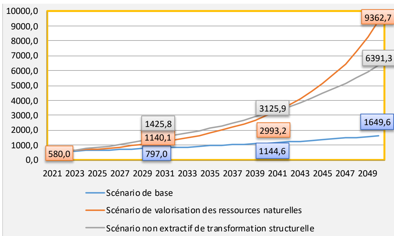
Figure 11. RDC, projections du RNDB par habitant (en dollars US constants de 2021) à l'horizon 2050 en trois scénarios
