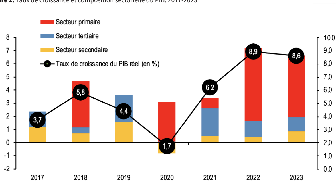
Figure 1. Taux de croissance et composition sectorielle du PIB, 2017-2023
