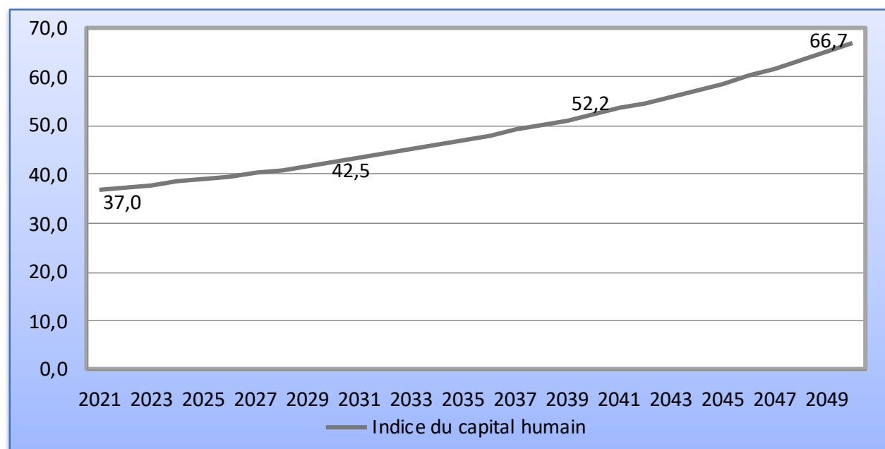
Figure 17. RDC, projections de l'indice du capital humain (échelle de 0 à 100, Banque Mondiale) à l'horizon 2050
