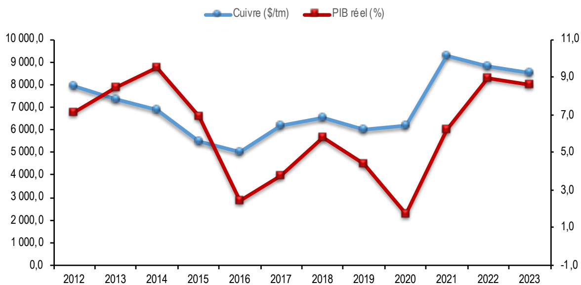
Figure 2. Évolution comparée du taux de croissance du PIB et du cours mondial du cuivre
