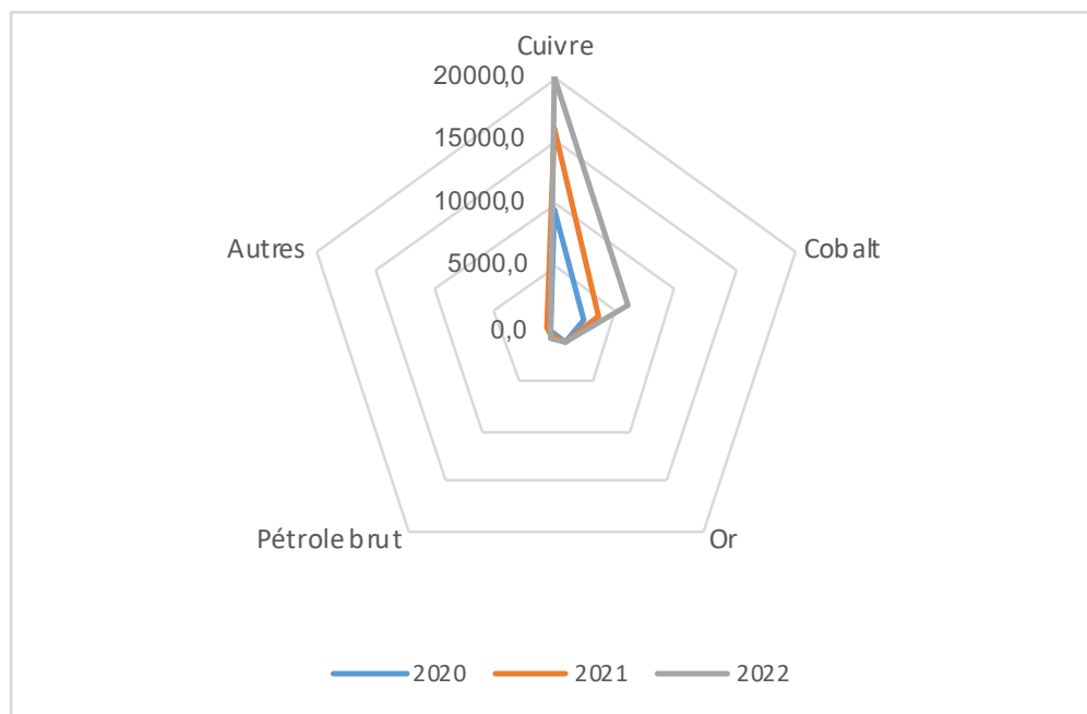
Figure 7. Composition sectorielle des exportations de la RDC, 2020-2022
